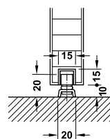
Floor guide with U-shaped guide track in door leaf and floor guide roller การติดตั้งกันแกว่งแบบ B
